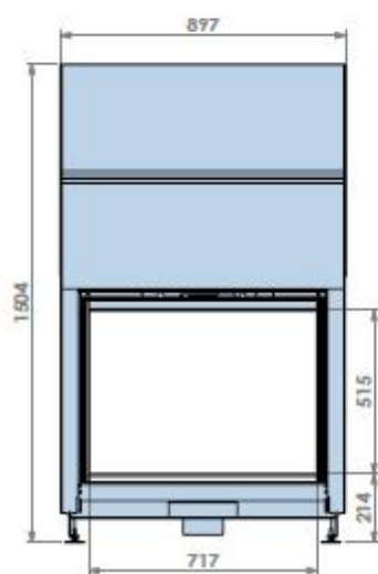
Voorraanzicht
