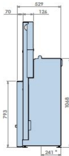
Zijaanzicht
