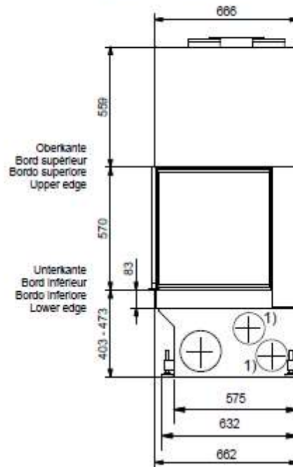
Seitenansicht / Vue de côté Vista laterale / Side view
