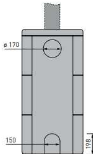
Rückansicht
