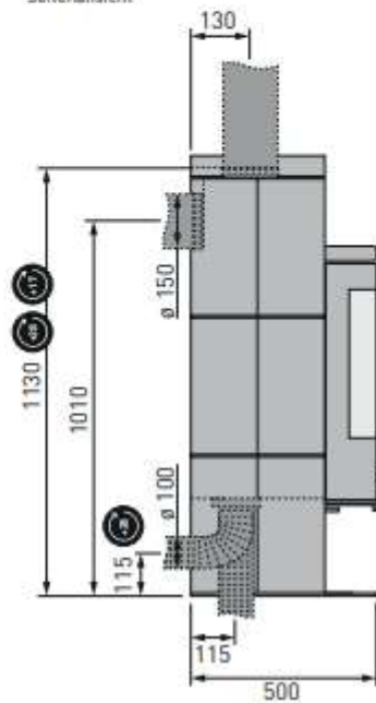
Seitenansicht
